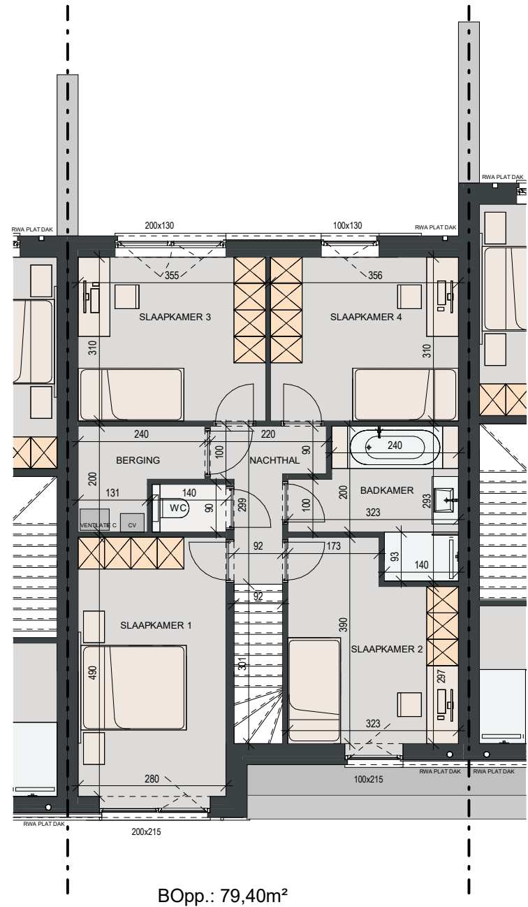
1e Verdieping 1:100
